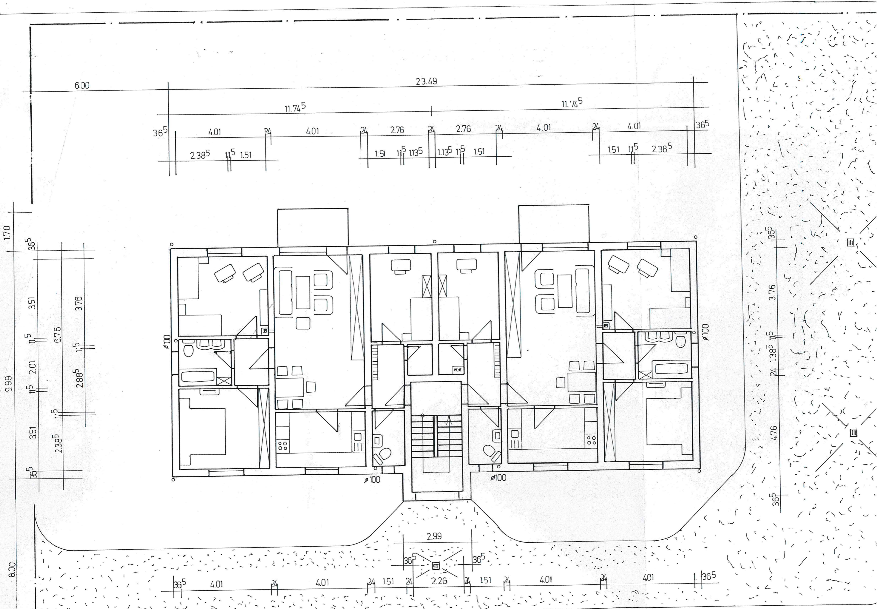
ERDGESCHOSS
